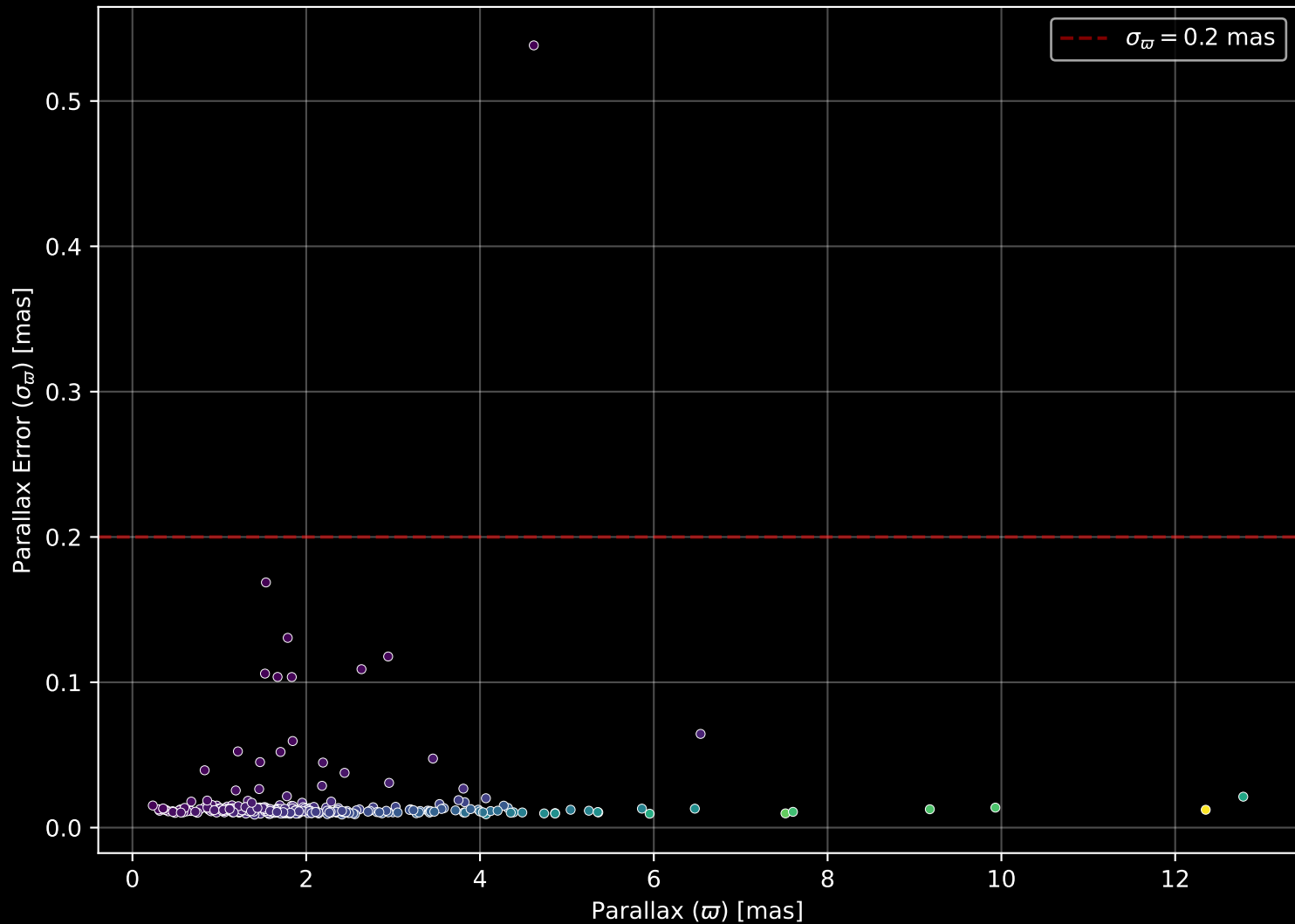
GALAH DR4 Field: [6858] Parallax Quality (n= 301)
