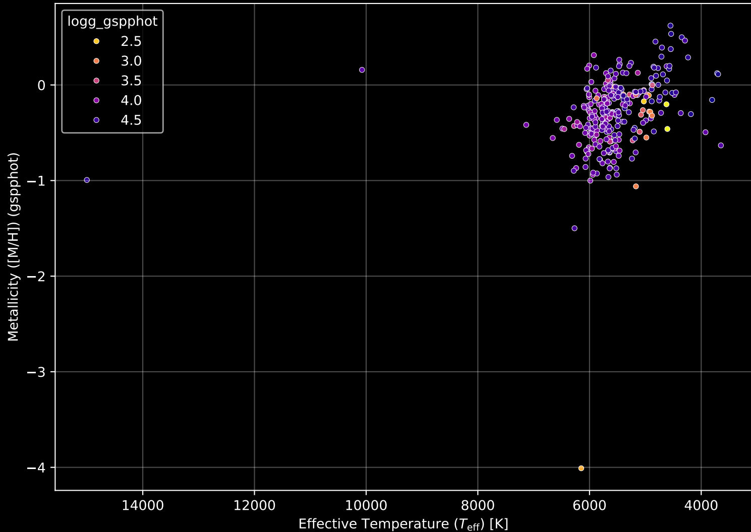
GALAH DR4 Field: [6858] Stellar Population Parameters (n= 301)
