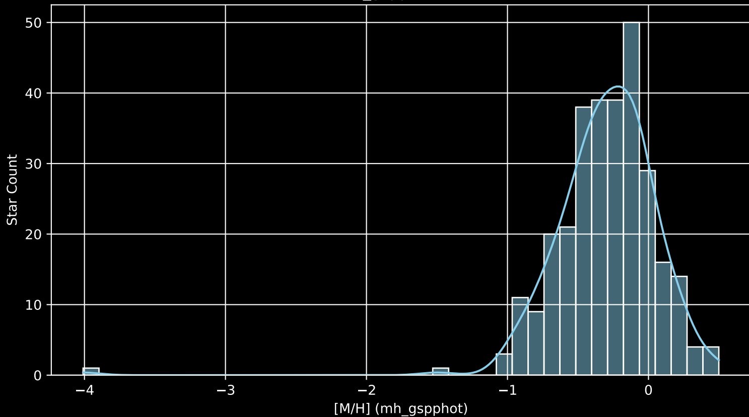
GALAH DR4 Field: [6858] [M/H] (mh_gspphot) (n= 299)
