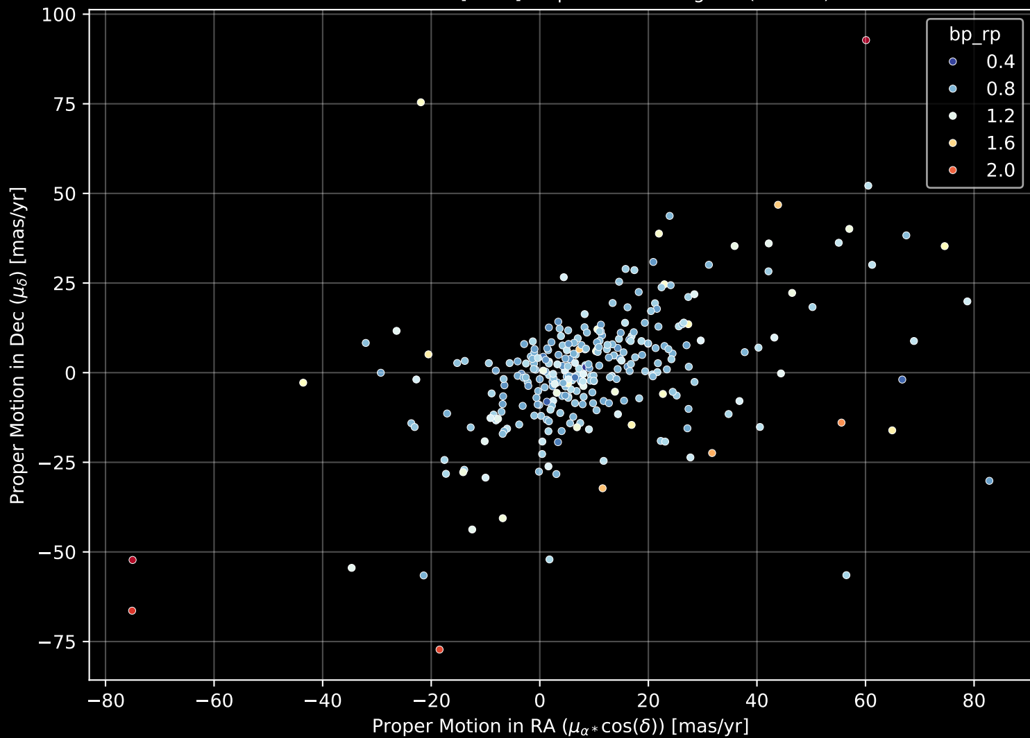
GALAH DR4 Field: [6858] Proper Motion Diagram (n= 301)
